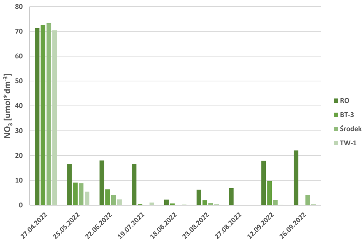
Rys. 5. Średnie stężenie \text{NO}_3 w wodach Zalewu Szczecińskiego i Rostki Odrzańskiej w całym sezonie wegetacyjnym 2022
