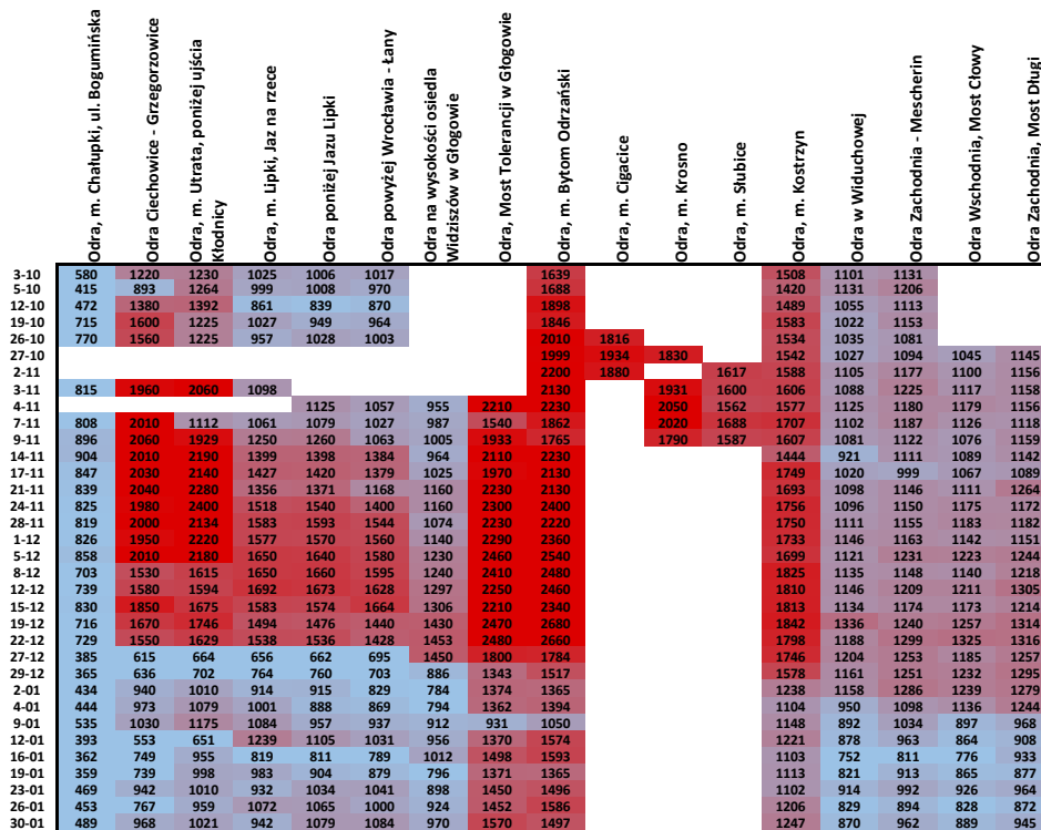
Rys. 6. Zmienność przestrzenna i czasowa przewodności elektrolitycznej właściwej ( \mu\text{S}/\text{cm} ) na stanowiskach monitoringu interwencyjnego na Odrze w okresie od października 2022 r. do końca stycznia 2023 r. Stanowiska uszeregowane wzdłuż biegu rzeki. Skala barwna: od <percyntyl 10% do >percyntyl 90%.
