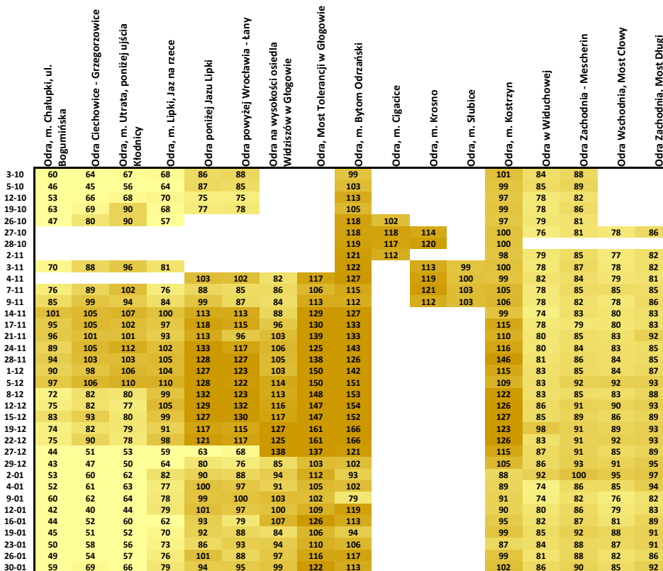
Rys. 8. Zmienność przestrzenna i czasowa stężenia siarczanów (mg/l) na stanowiskach monitoringu interwencyjnego na Odrze od października 2022 r. do końca stycznia 2023 r. Stanowiska uszeregowane wzdłuż biegu rzeki. Skala barwna: od <percytyl 10% do >percytyl 90%.
