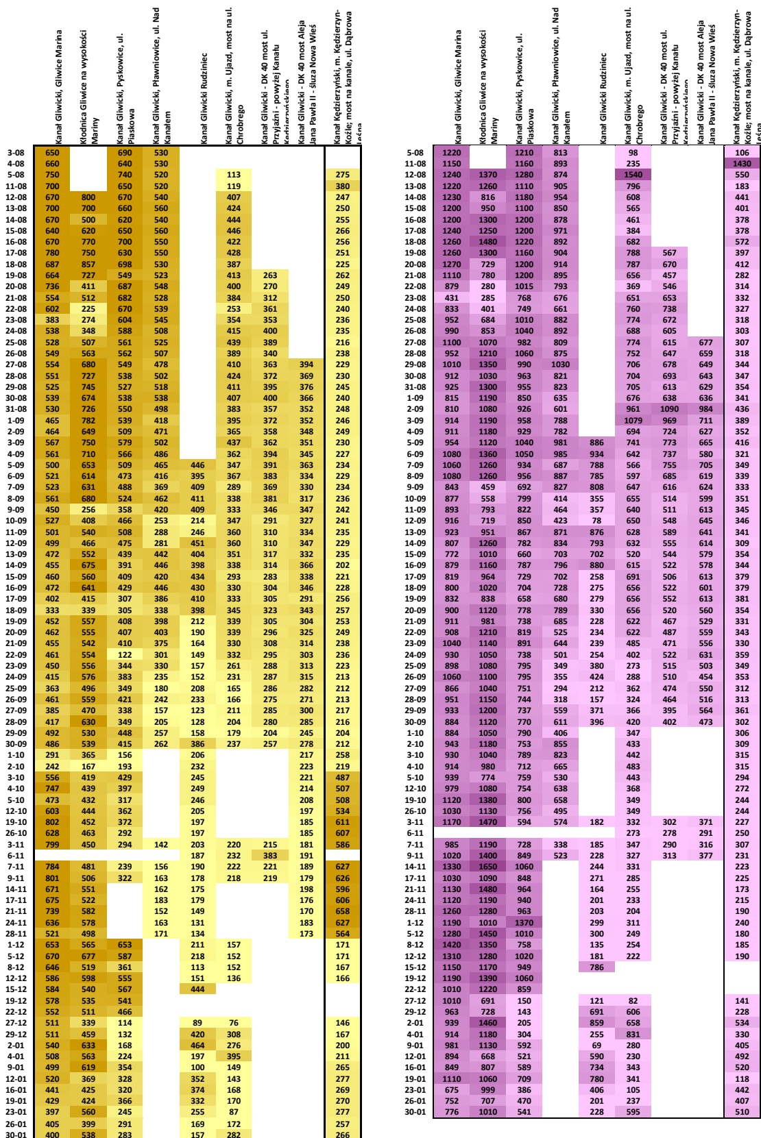
Rys. 11. Zmienność przestrzenna i czasowa stężenia siarczanów (mg/l) i sodu (mg/L) na poszczególnych stanowiskach monitoringu interwencyjnego na Kanale Gliwickim, rzecze Kłodnicy i Kanale Kędzierzyn-Koźle w okresie od sierpnia 2022 r. do końca stycznia 2023 r. Stanowiska uszeregowane począwszy od górnego biegu rzeki od strony lewej. Skala barwna: od < percentyl 10% do >percentyl 90%.
