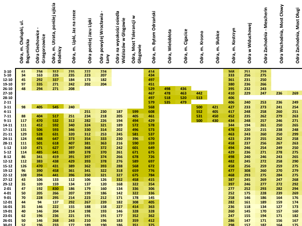
Rys. 7. Zmienność przestrzenna i czasowa stężenia chlorków ( \text{mg}/\text{l} ) na stanowiskach monitoringu interwencyjnego na Odrze i Zalewie Szczecińskim w okresie od października 2022 r. do końca stycznia 2023 r. Stanowiska uszeregowane wzdłuż biegu rzeki. Skala barwna: od <percyntyl 10% do >percyntyl 90%.
