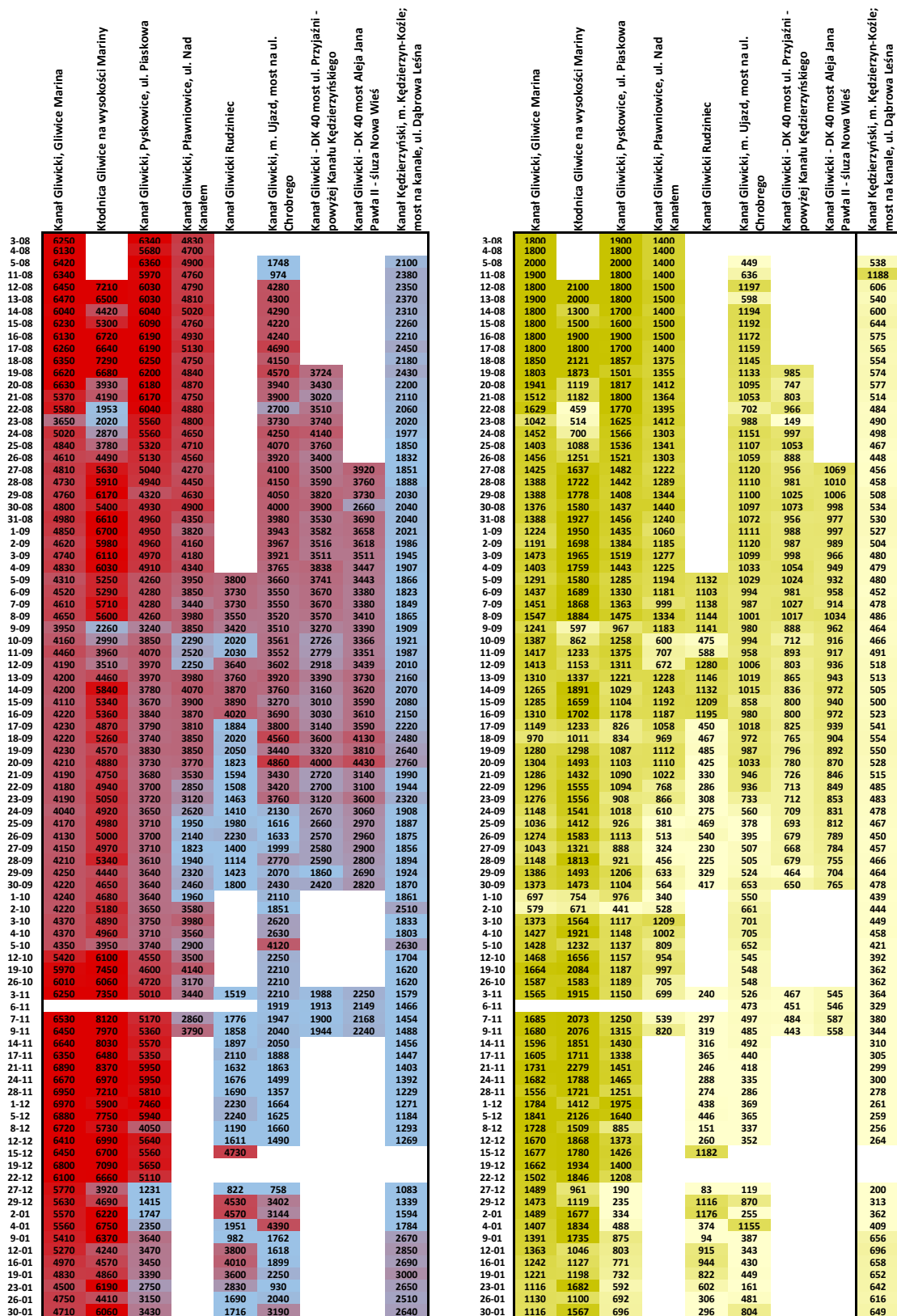
Rys. 10. Zmienność przestrzenna i czasowa przewodności elektrolitycznej właściwej ( \mu\text{S/cm} ) – lewy panel oraz chlorków ( \text{mg/l} ) - prawy panel na stanowiskach monitoringu interwencyjnego na Kanale Gliwickim, rzece Kłodnicy i Kanale Kędzierzyn-Koźle w okresie od sierpnia 2022 r. do końca stycznia 2023 r. Stanowiska uszeregowane wzdłuż biegu rzeki. Skala barwna: od <percentyl 10% do >percentyl 90%.
